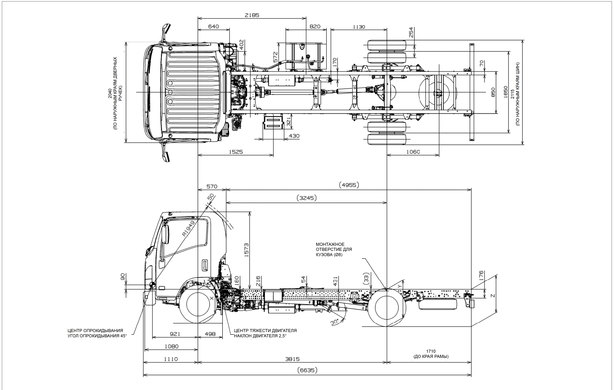
Рис. 9-1-5. Чертеж шасси с кабиной. NPR75L-KL5VAYUN
